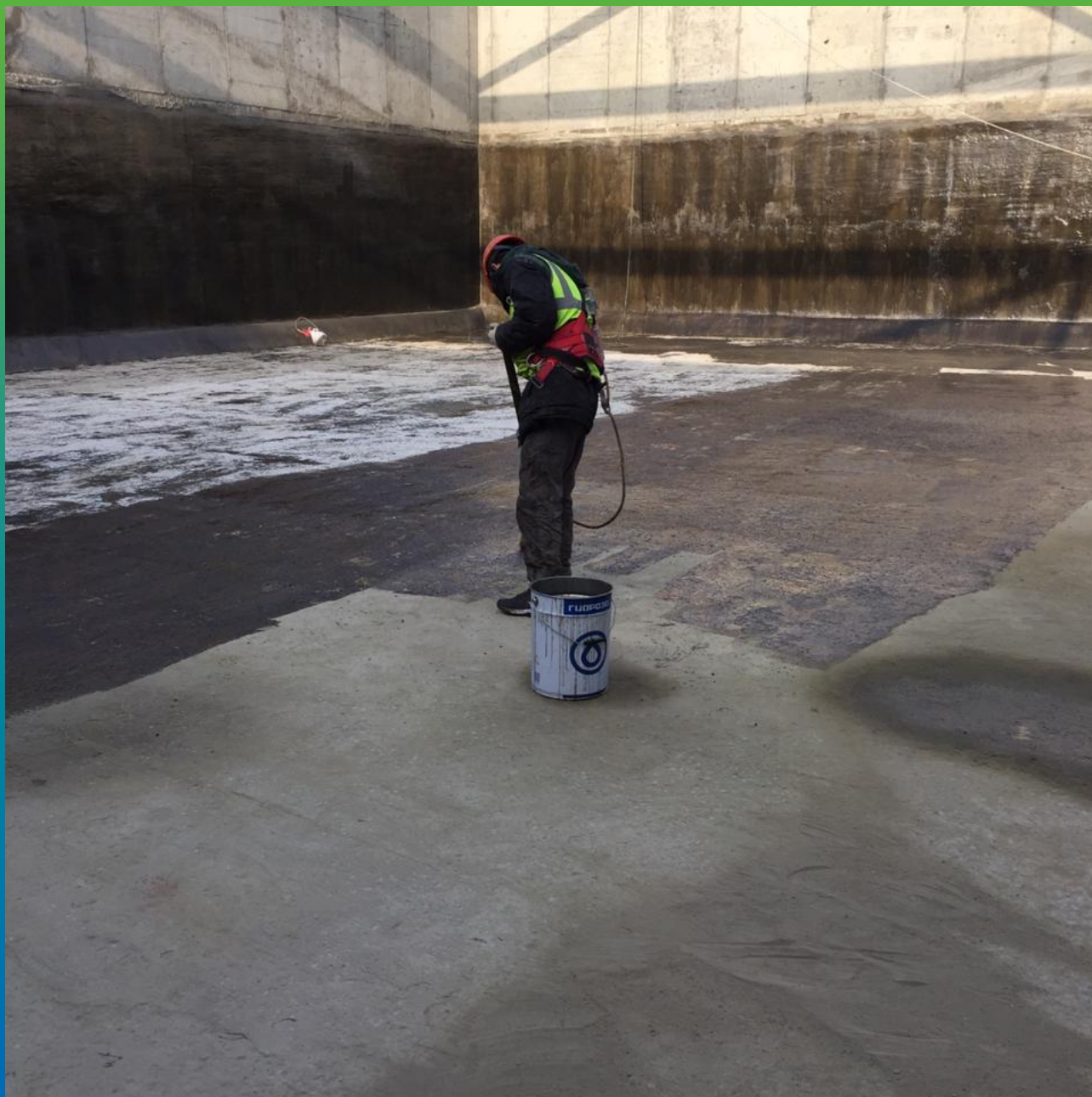
Нанесение эпоксидной грунтовки ДенТоп ЭП 100 на днище резервуара
