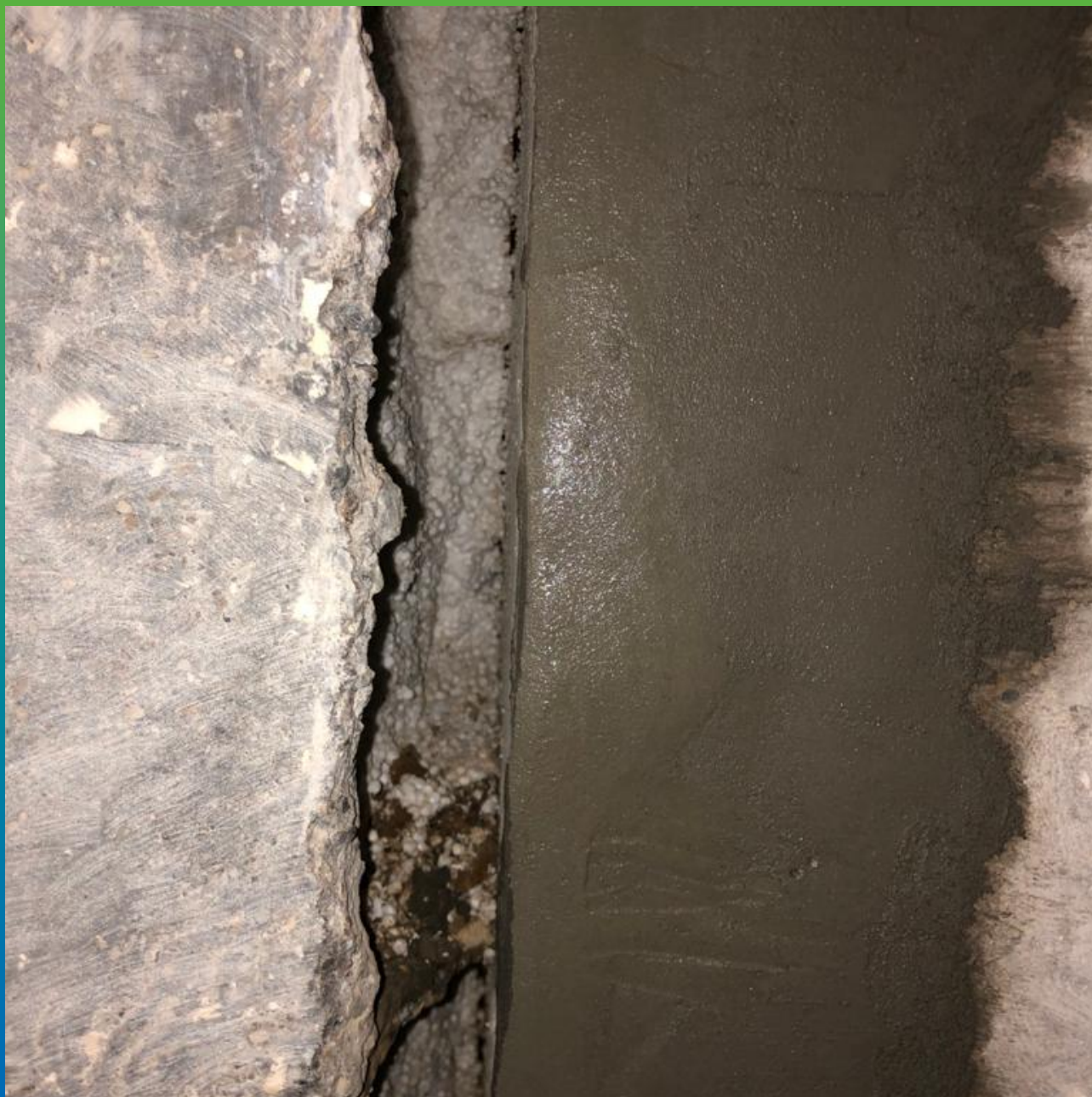
Кромки шва, восстановленные составом Стармекс РМ 3
