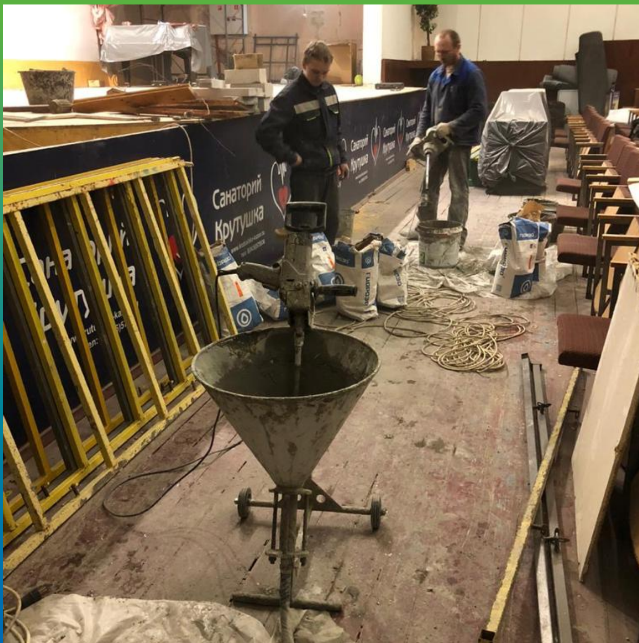
Шнековый насос, готовый к производству работ.
