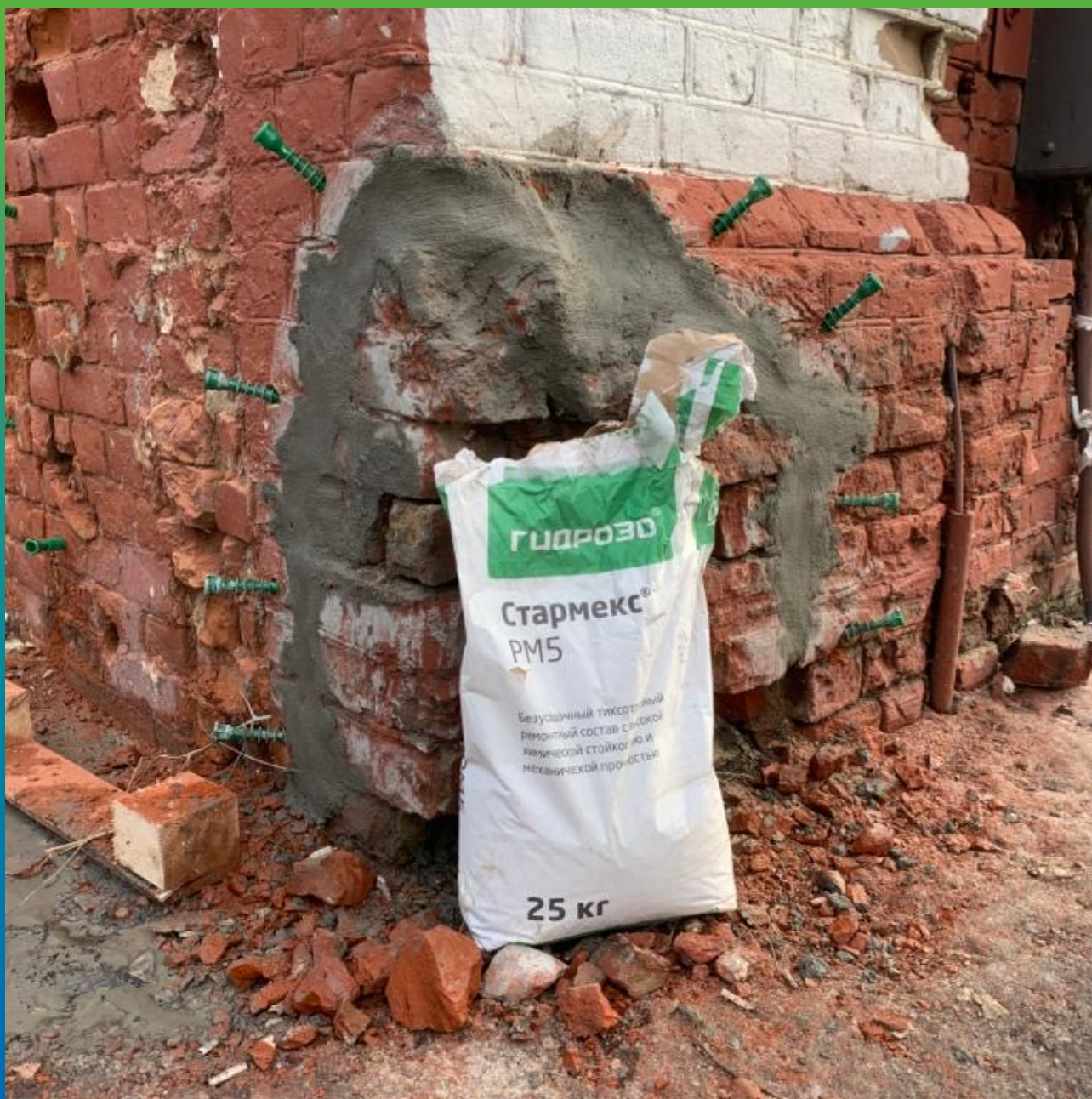
Трещина, зачеканенная составом Стармекс PM5
