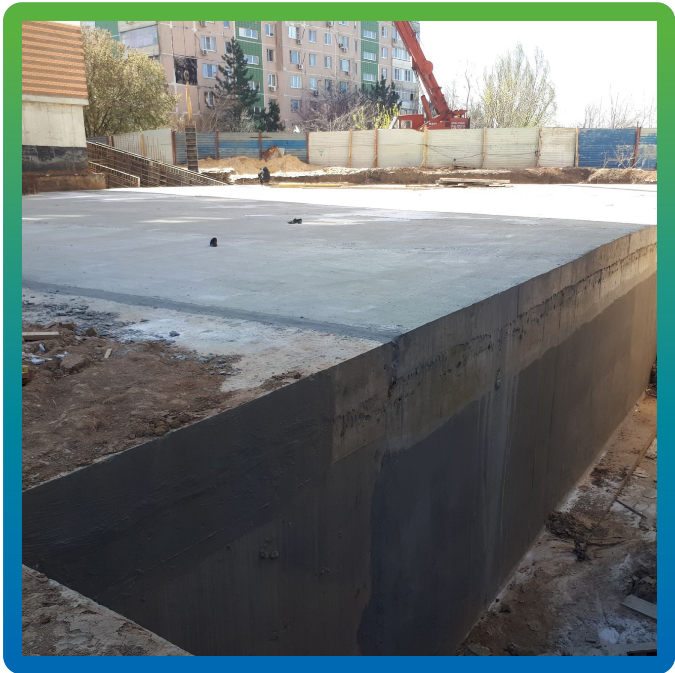
В процессе покрытия стен Стармекс Сил Флекс
