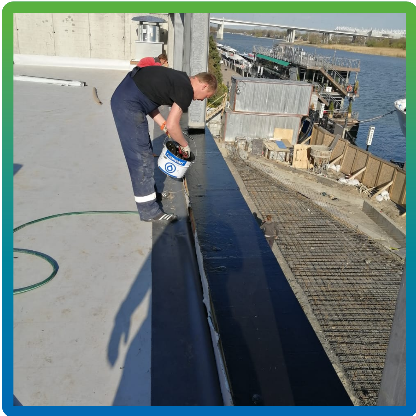
Нанесение полисульфидного покрытия ДенсТоп ПС 391
