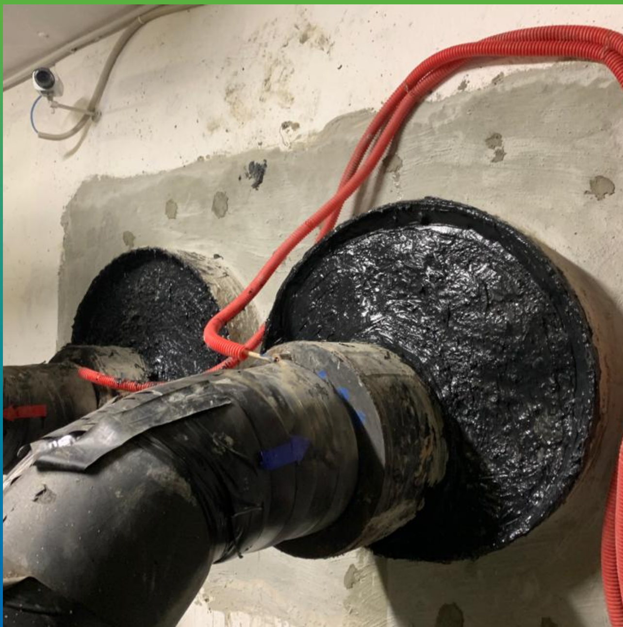
Герметизация ввода коммуникаций герметиком Манодил Бонд Ф
