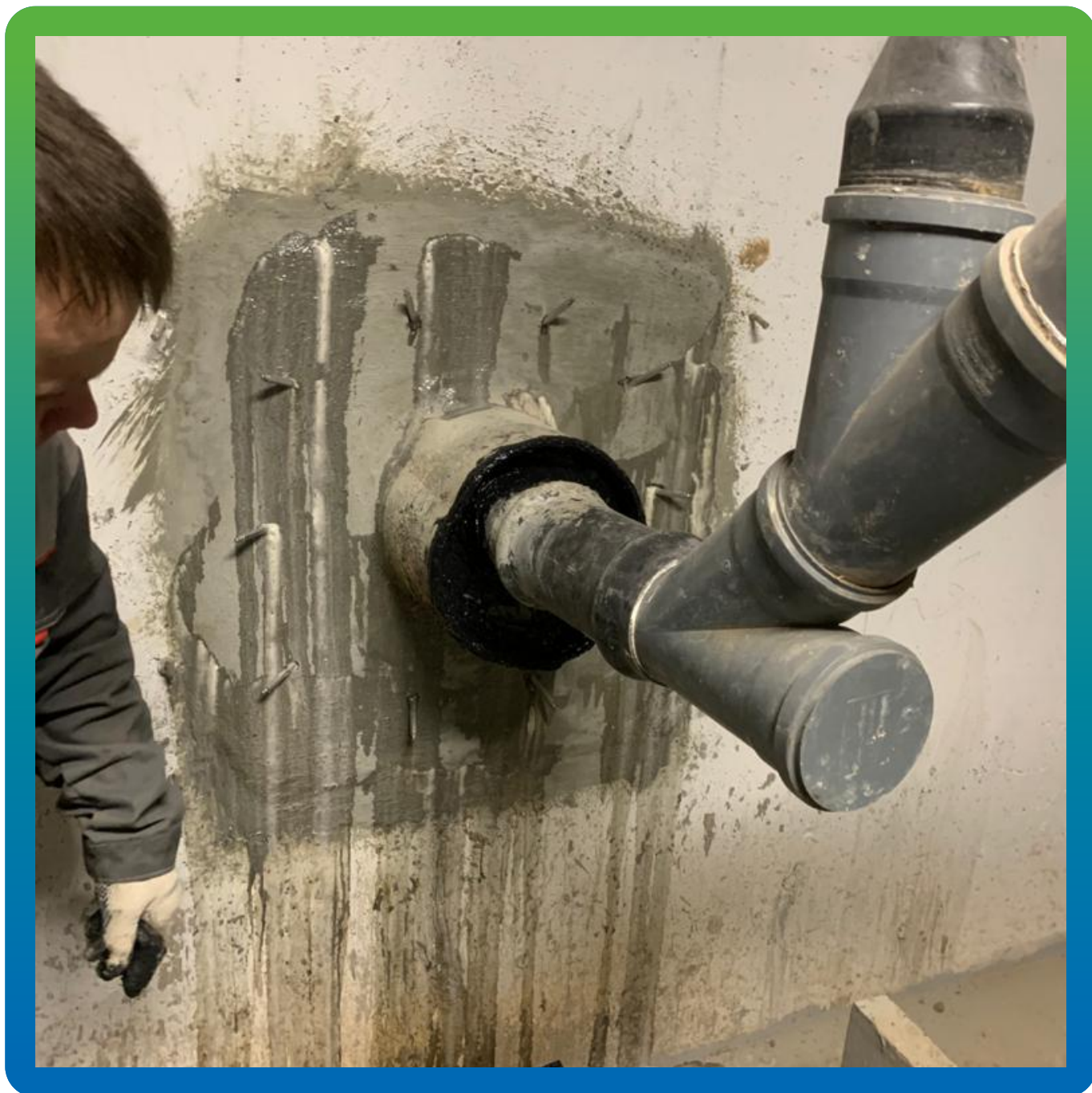
Инъектирование полиуретановым составом Манопур С
