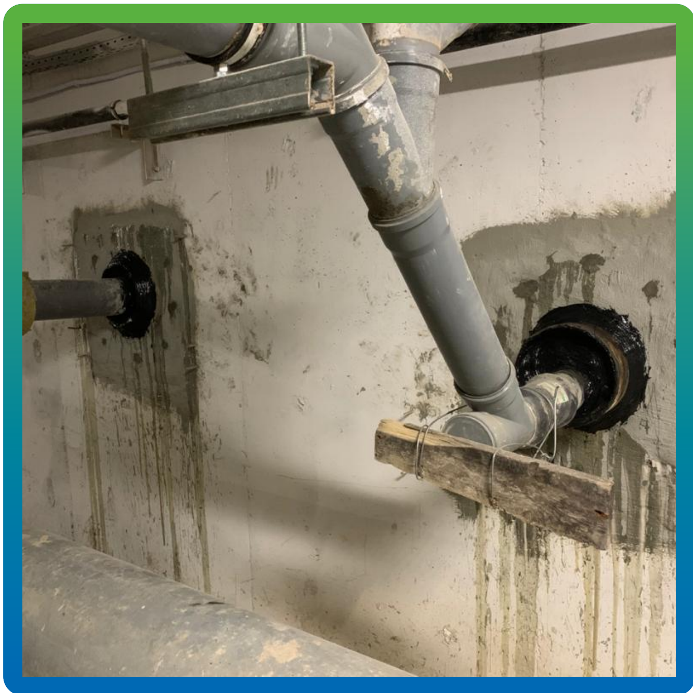
Герметизация ввода коммуникаций герметиком Манодил Бонд Ф
