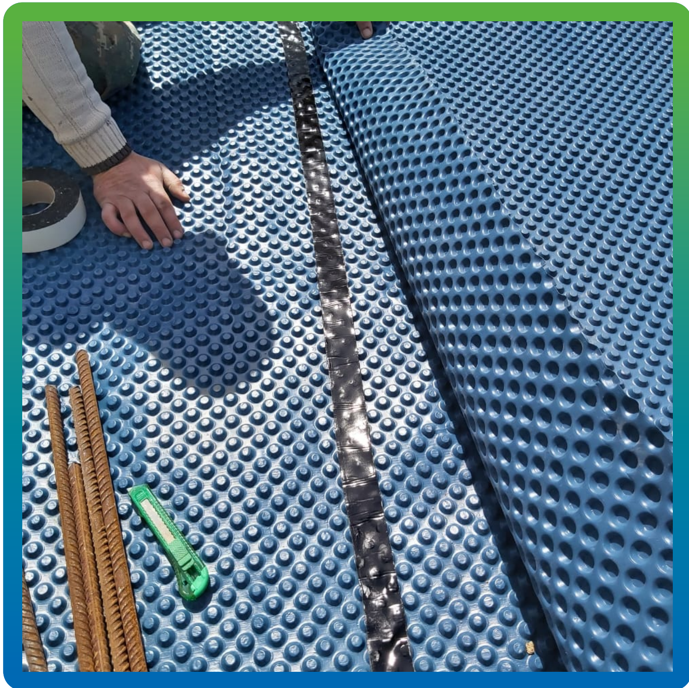
Скрепление мембраны Максдрейн 8 между собой
