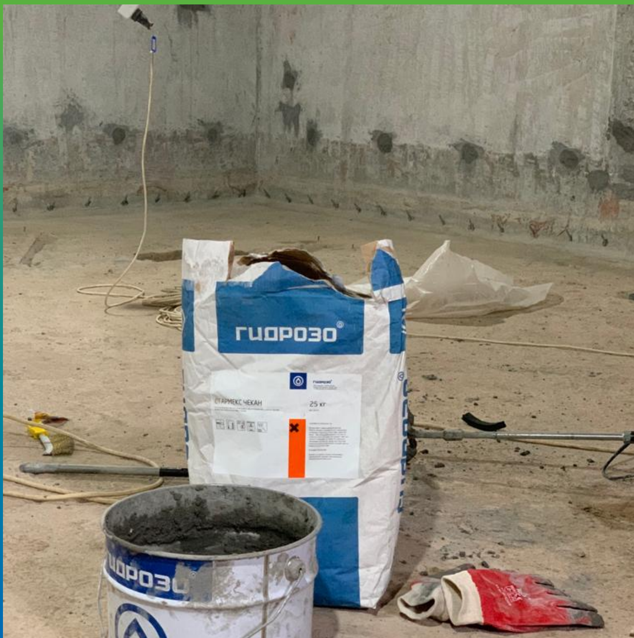
Зачеканка опалубочных отверстий составом Стармекс Чекан
