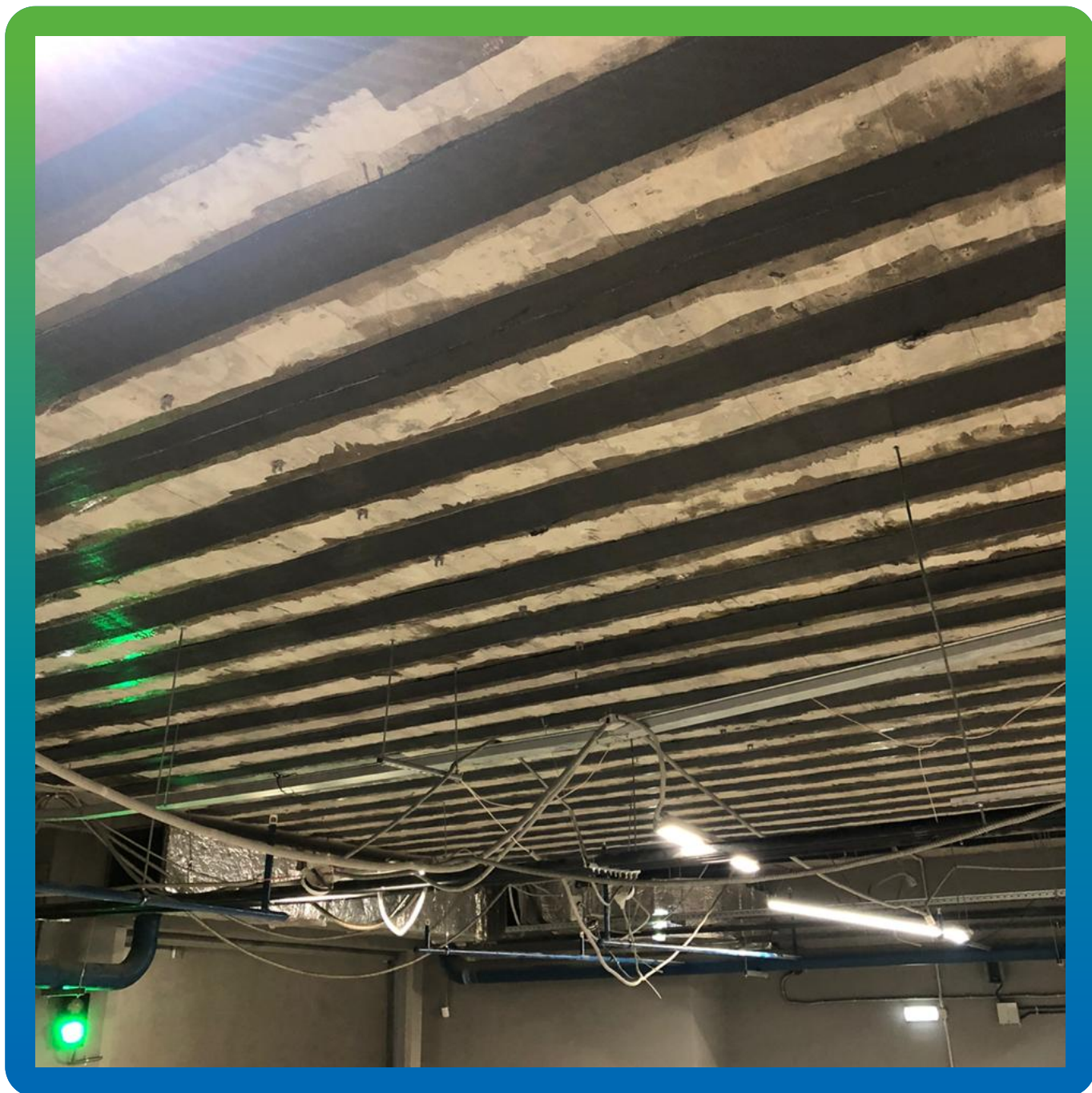
Монтаж системы Армошел
