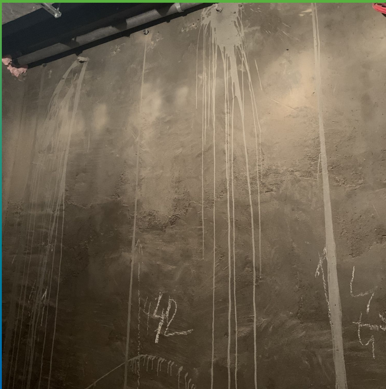
Стены, проинъектированные Маноцем Гроут
