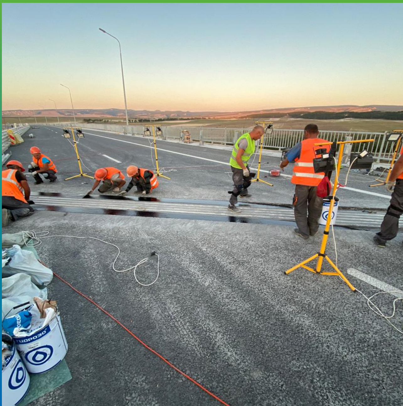
Выравнивание уложенного состава в штробу
