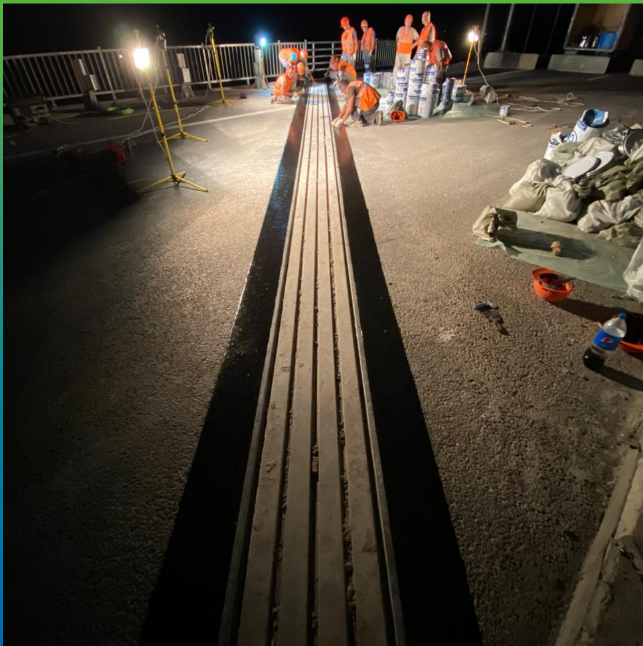
Завершение работ по укладке состава Манопур 336 в переходную зону деформационного шва.
