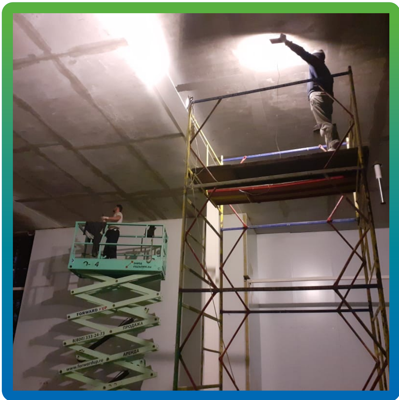
Нанесение грунтовочного состава ДенсТоп ЭП 106 на перекрытие
