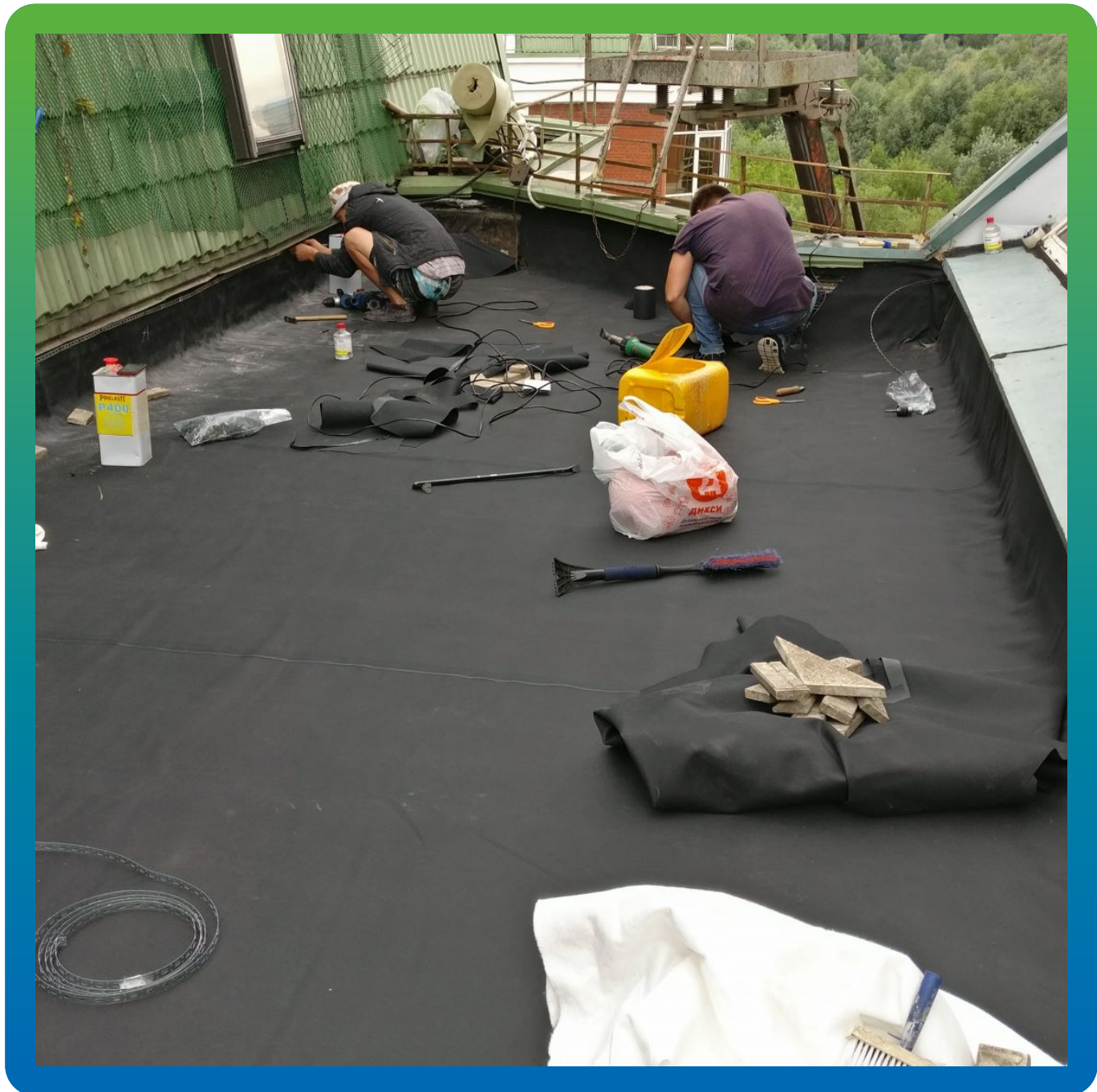
Обварка углов и закрепление краевой рейкой
