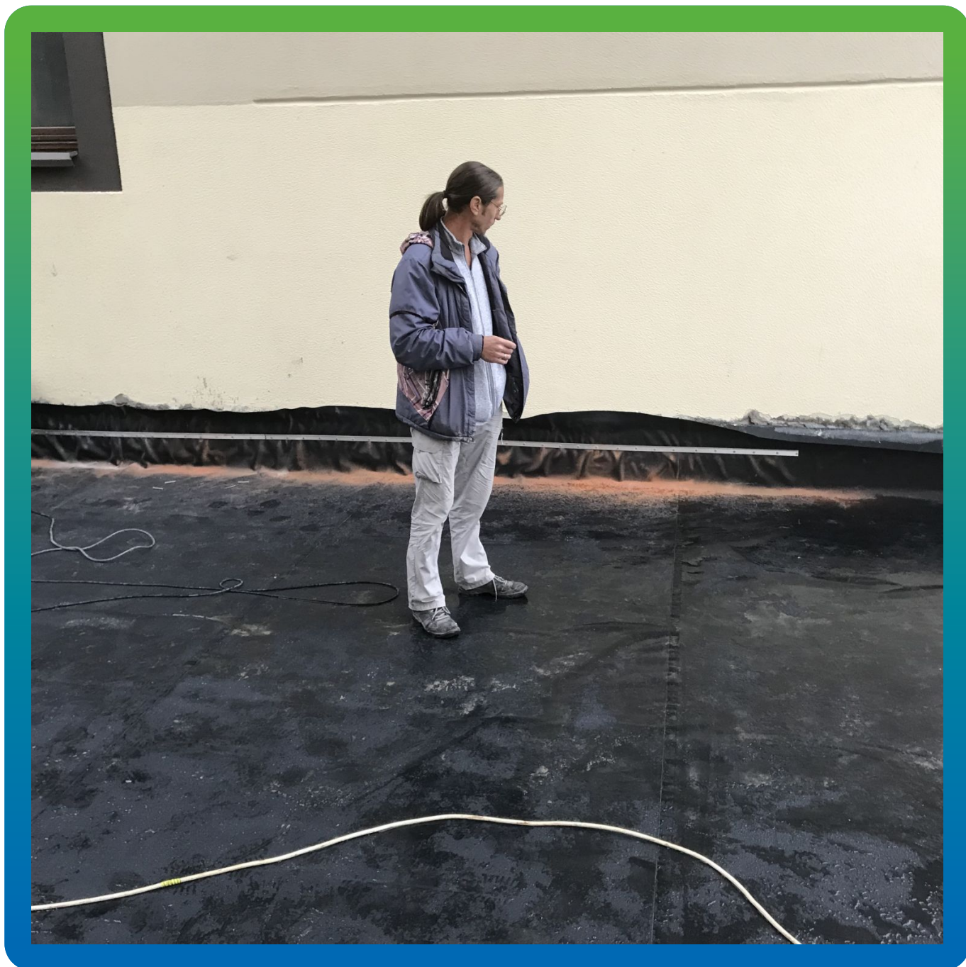
Крепление краевой рейкой к вертикальному основанию
