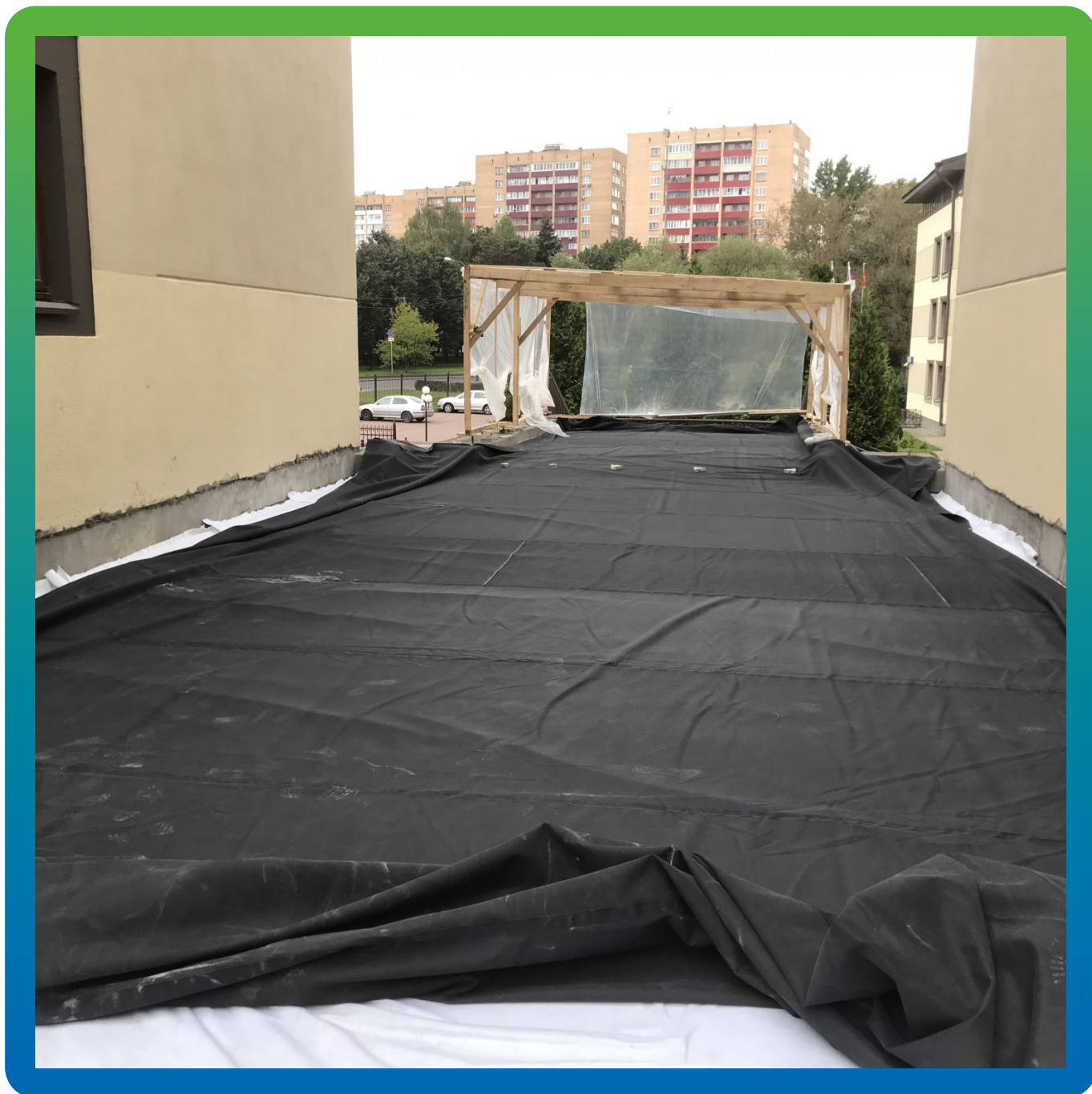
Раскатка мембраны по всей площади основания
