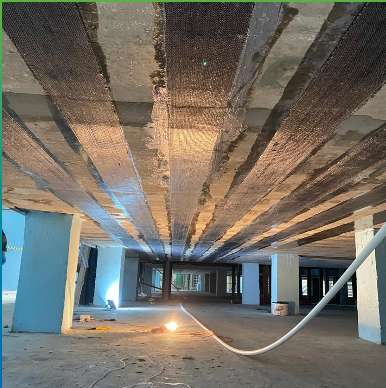
Монтаж КСУ в продольном направлении, первый слой
