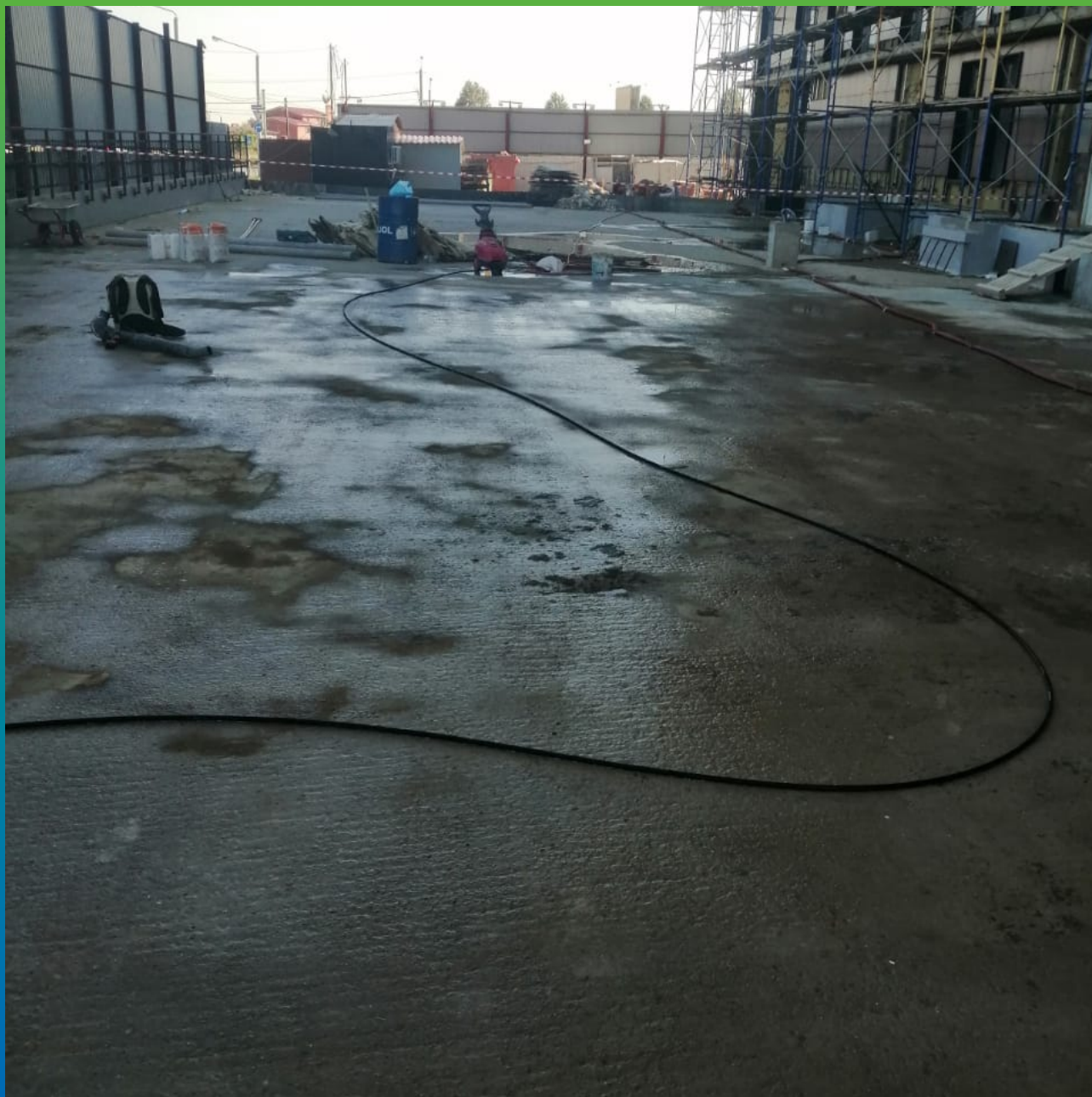
Увлажнение бетона эксплуатируемой кровли перед нанесением гидроизоляции
