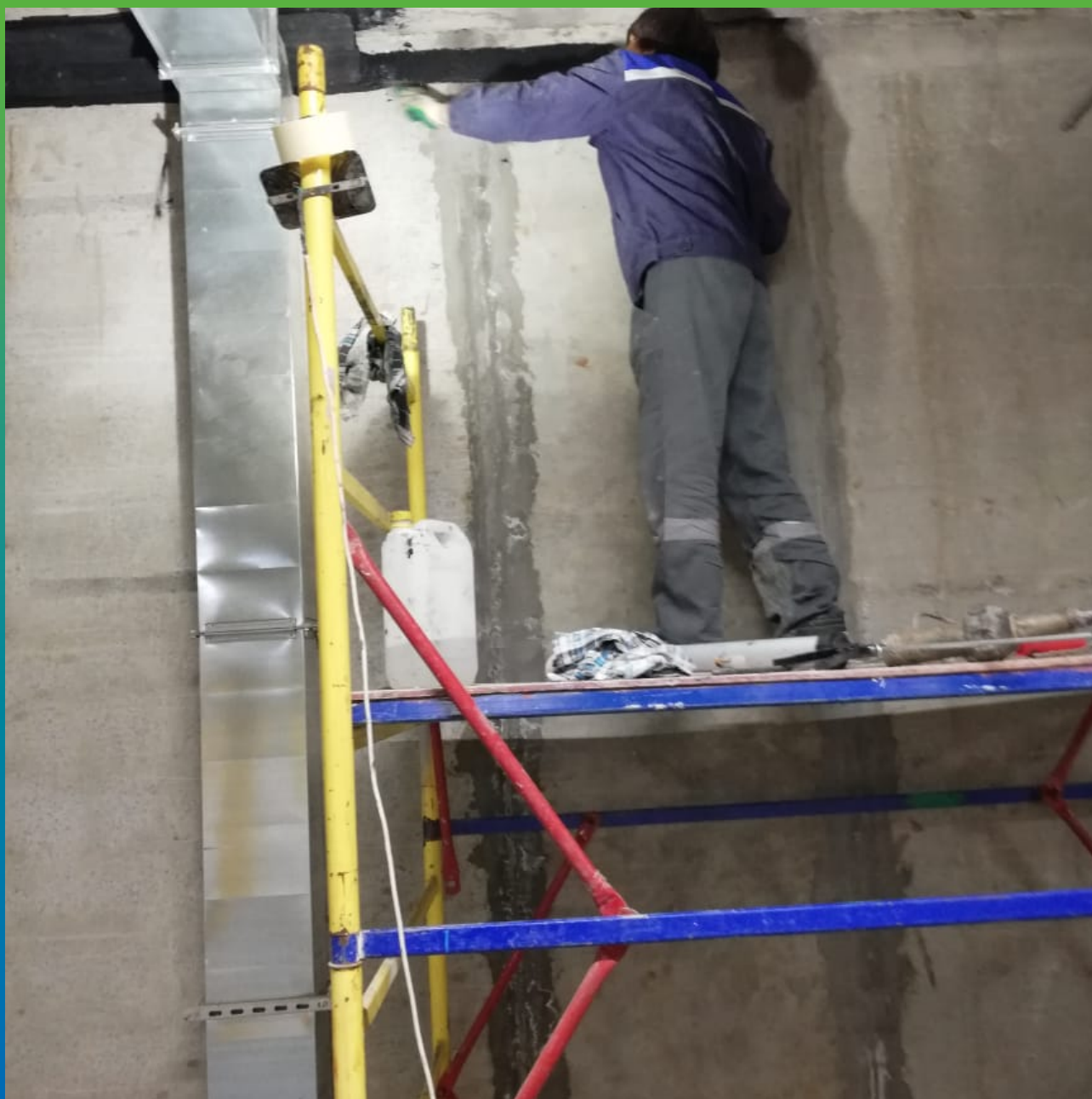
Монтаж ленты Преласты СТ
