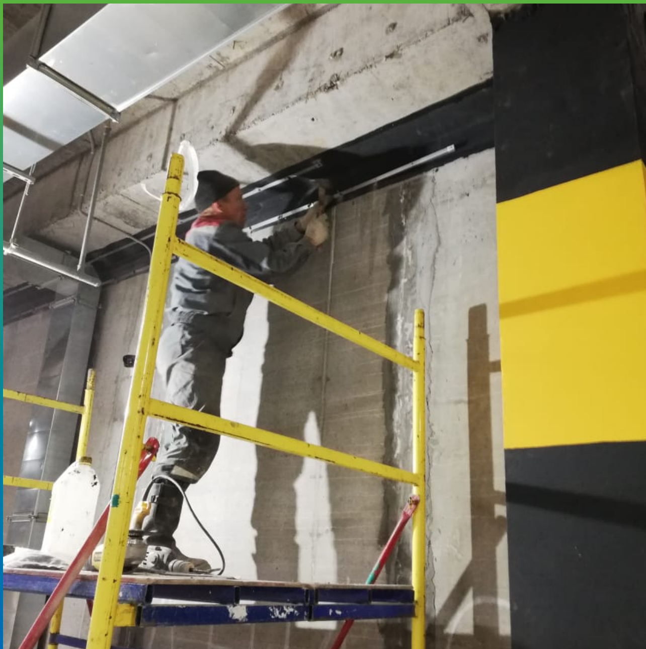
Крепление прижимной планки
