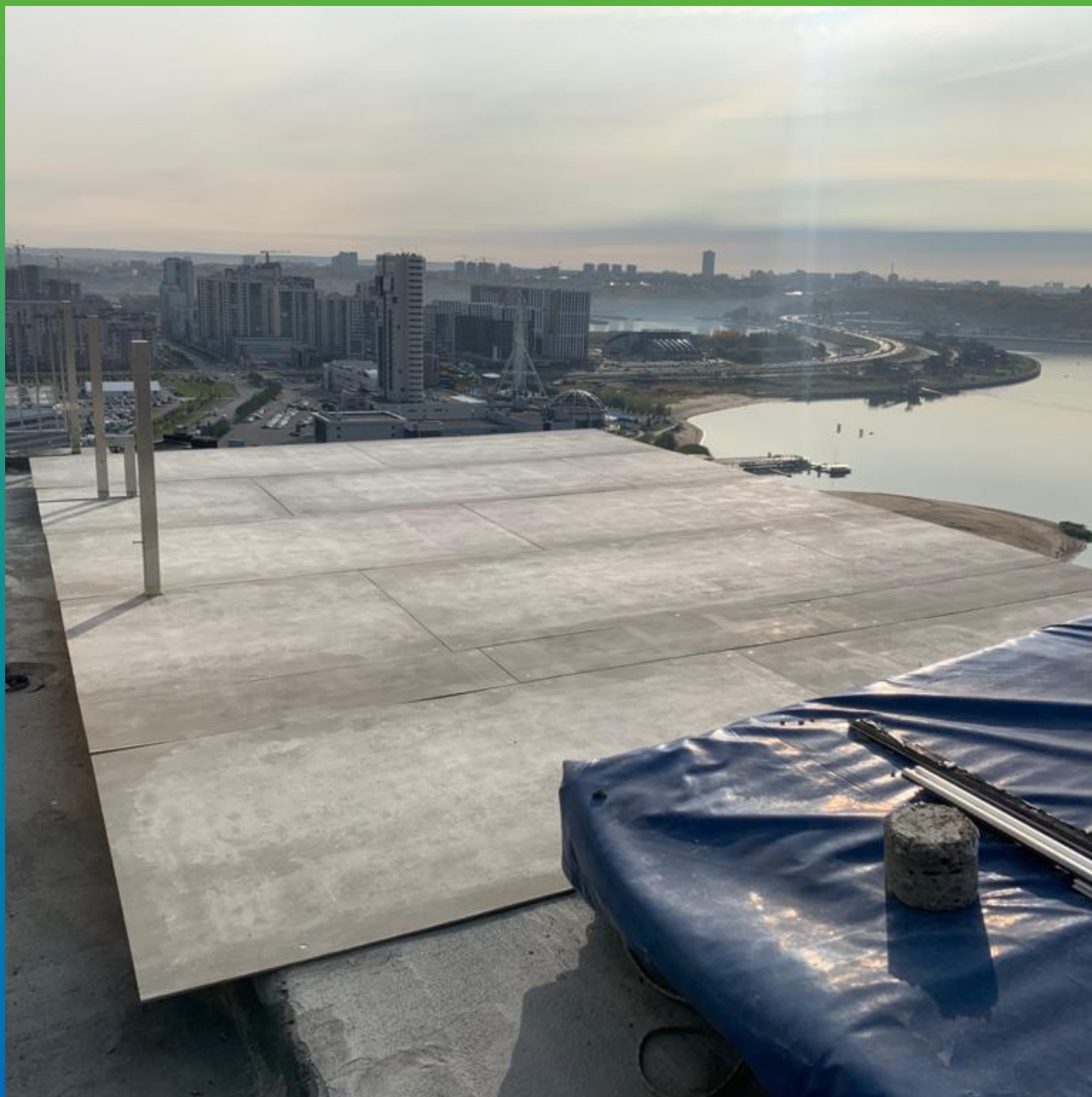
Основание из ЦСП под нанесение гидроизоляционного материала
