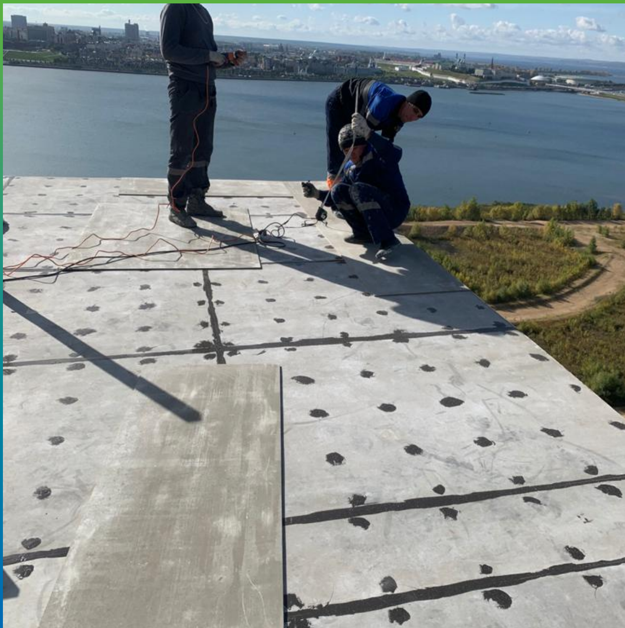
Герметизация стыков и монтажных отверстий герметиком Манодил Бонд Ф
