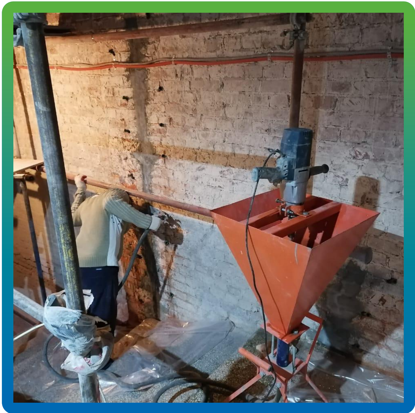
Инъекционные работы
