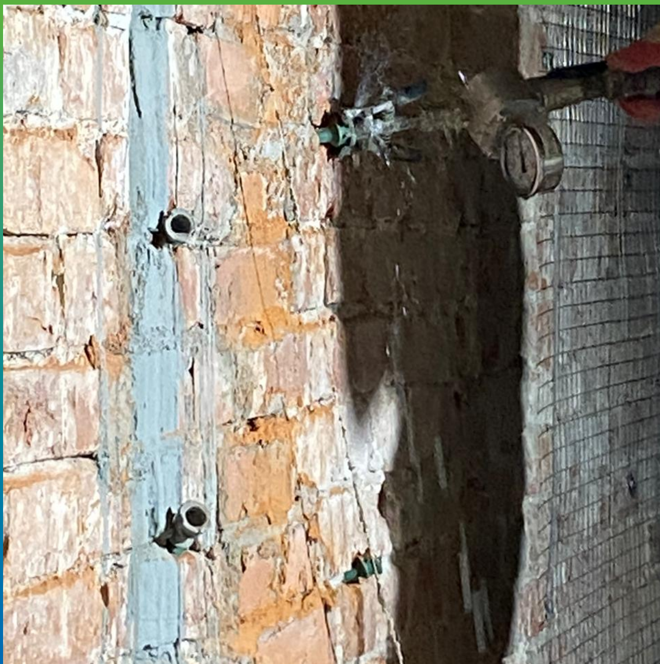
Прокачка материала Маноцем Фил в стену
