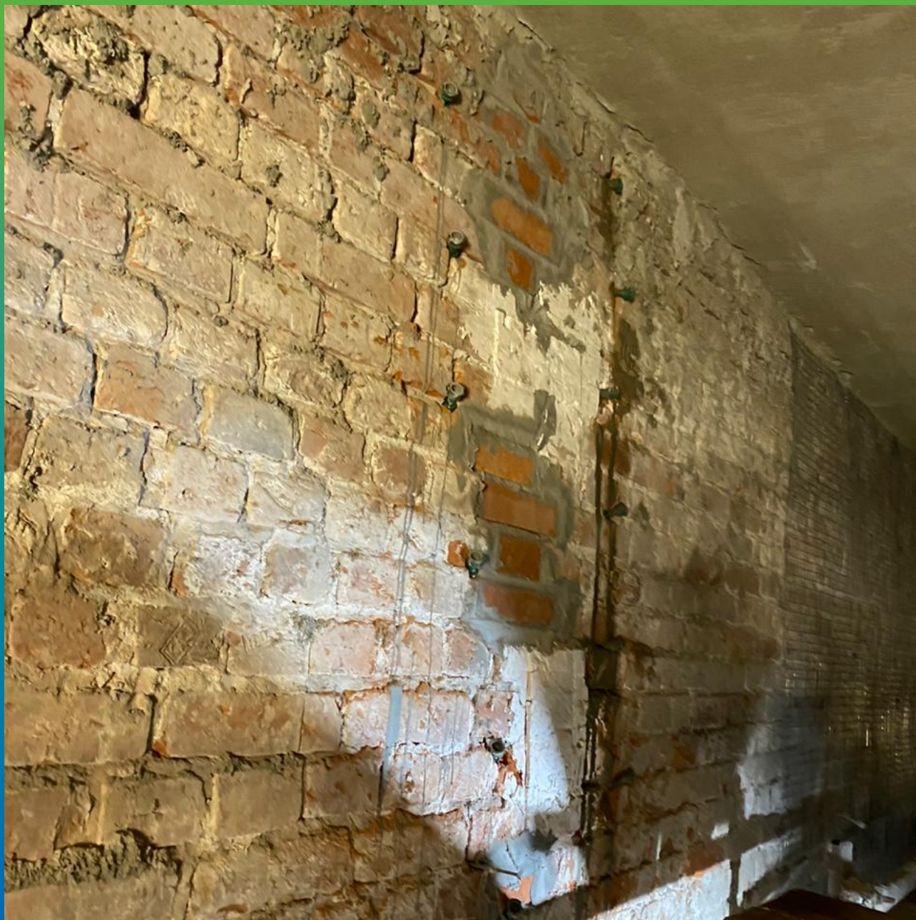
Установка пакеров с ламельной головкой для прокачки материала
