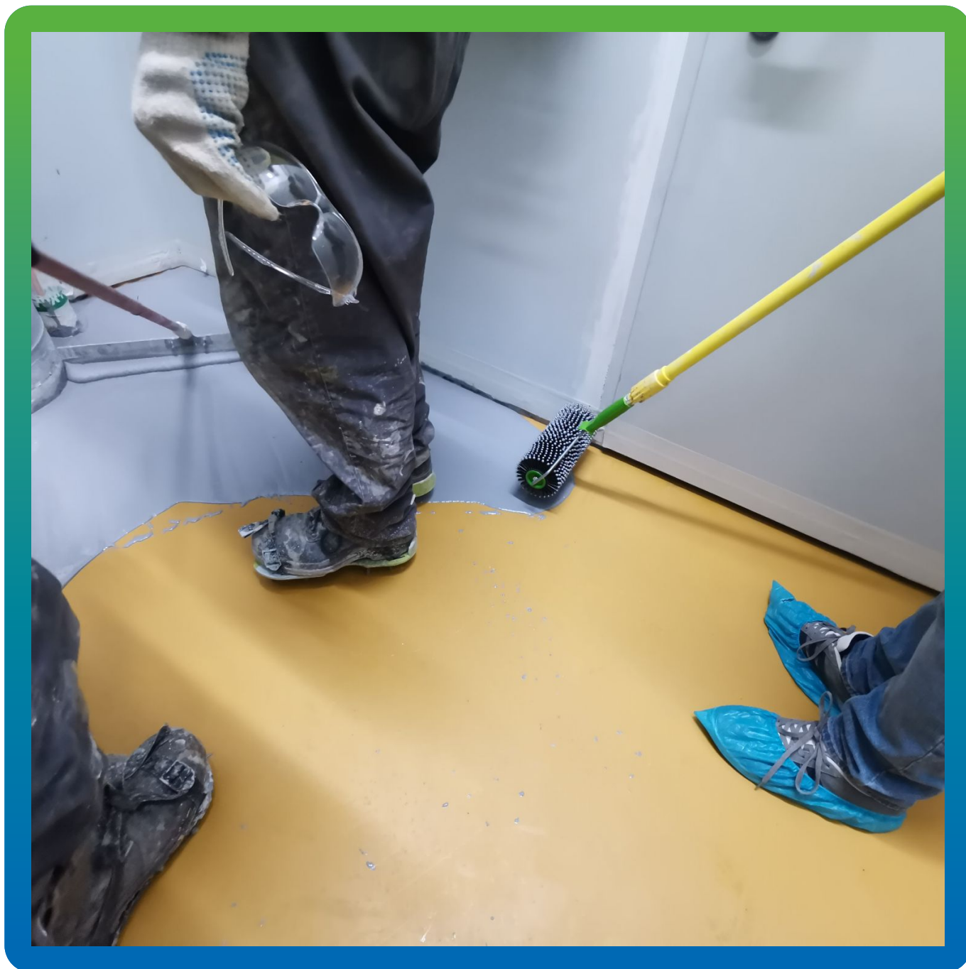
Удаление воздуха из покрытия с помощью игольчатого валика
