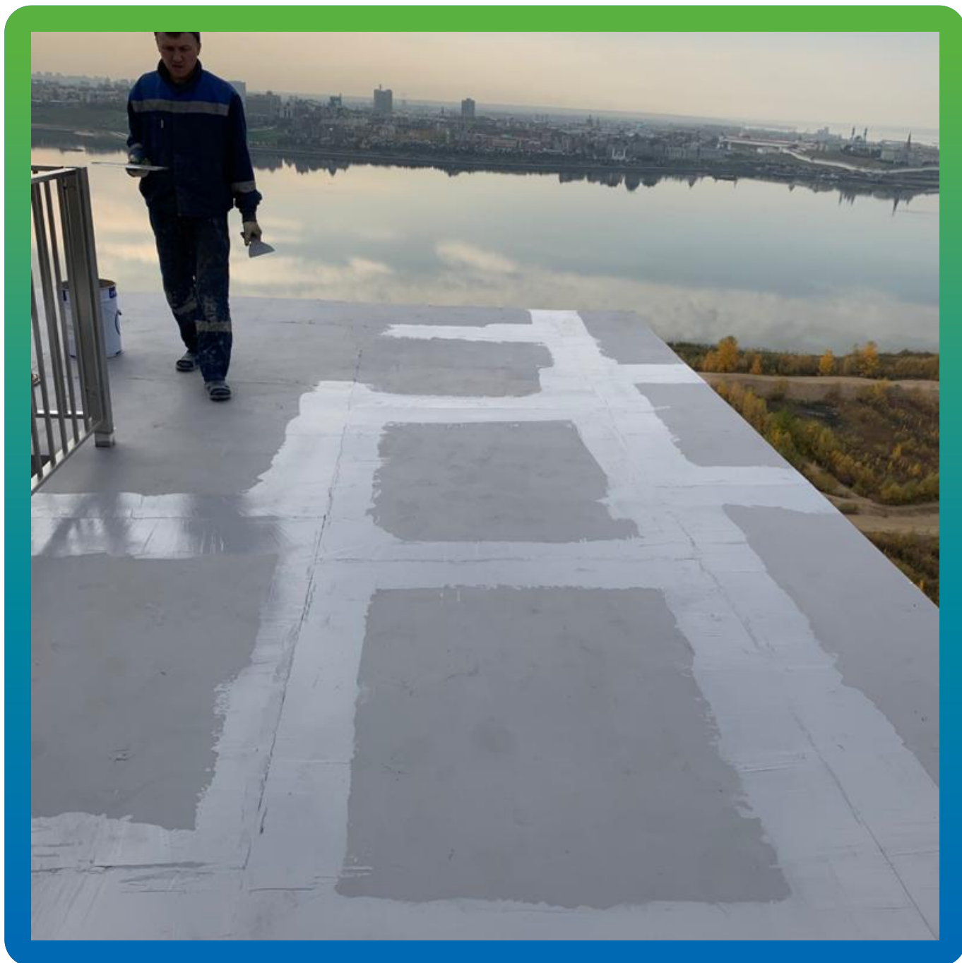
Грунтование составом ДенТоп ЭП 105
