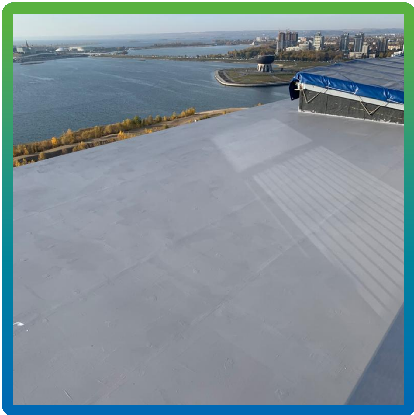
Грунтовочный состав ДенТоп ЭП 105, нанесенный на поверхность ЦСП плит
