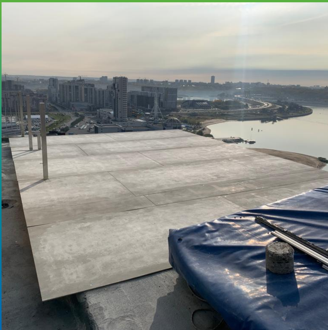
Подготовка выступающей террасы для нанесения Денстоп ПУ 325 Аква. Укладка ЦСП плит
