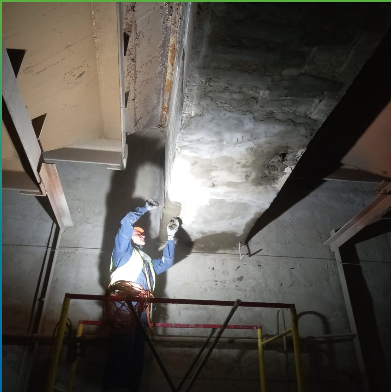
Нанесение состава Стармекс РМЗ для конструкционного ремонта бетона
