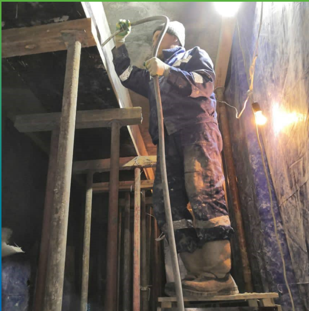
Инъектирование состава Маноцем Гроут в опалубку
