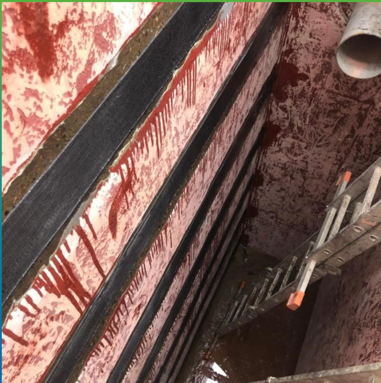
Армошел KB 500, монтированный на внутреннюю поверхность резервуара как дополнительное армирование
