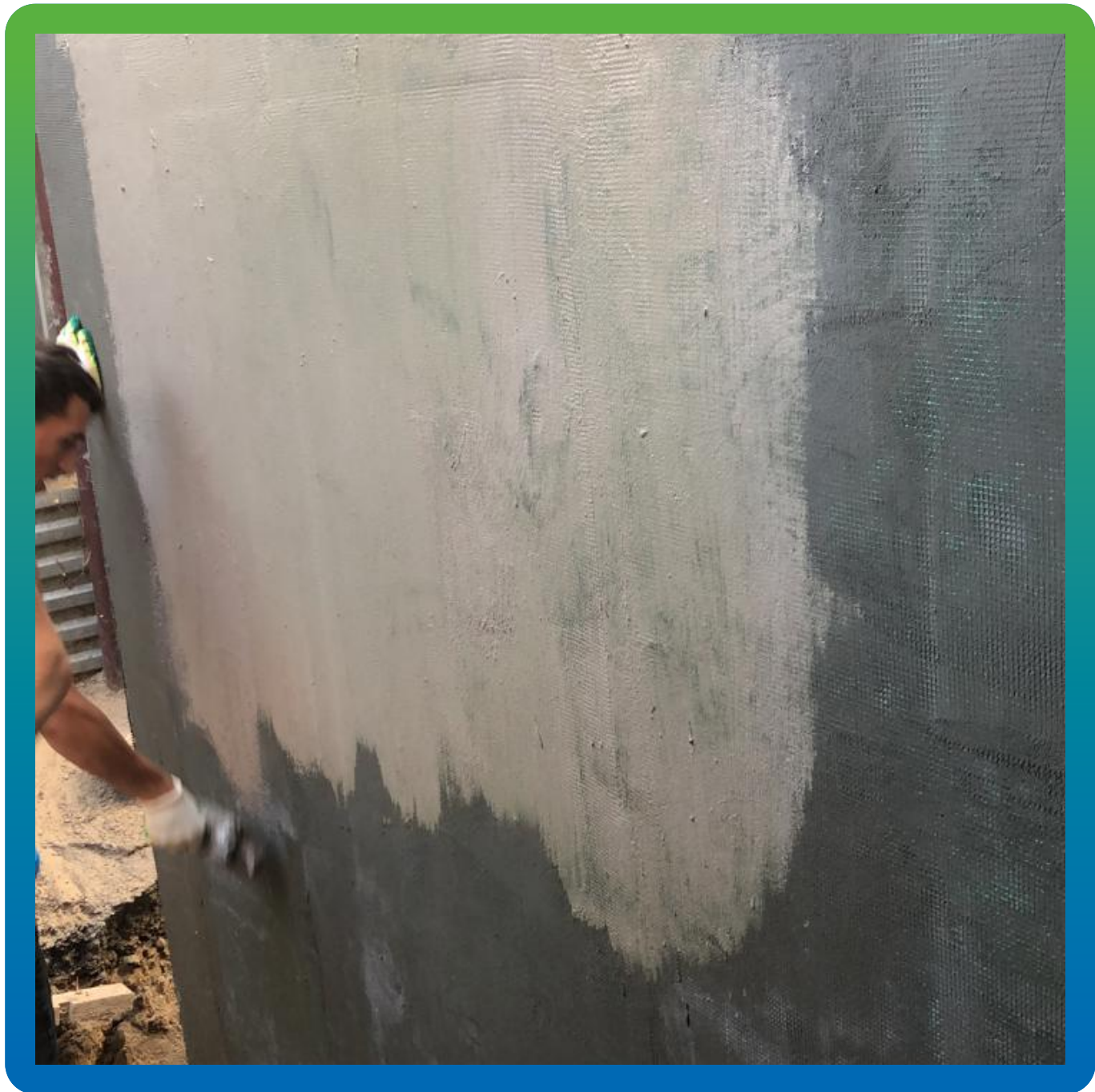
Нанесение второго слоя гидроизоляции по сетке.
