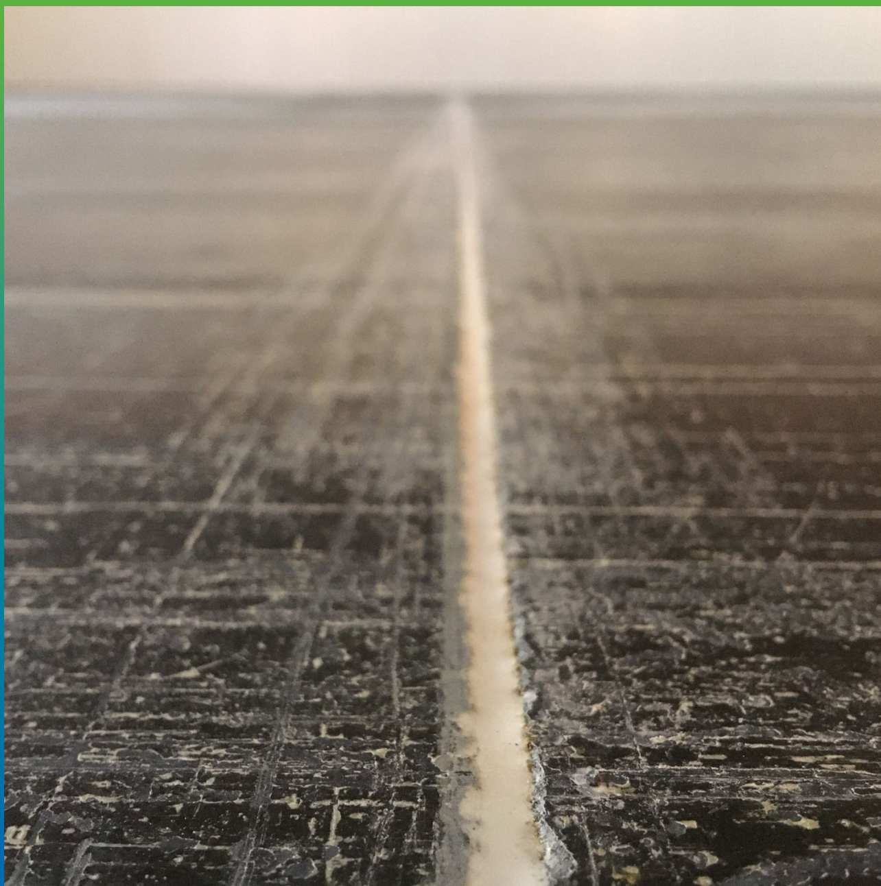
Шов заполненный герметиком Манодил ПУ 696
