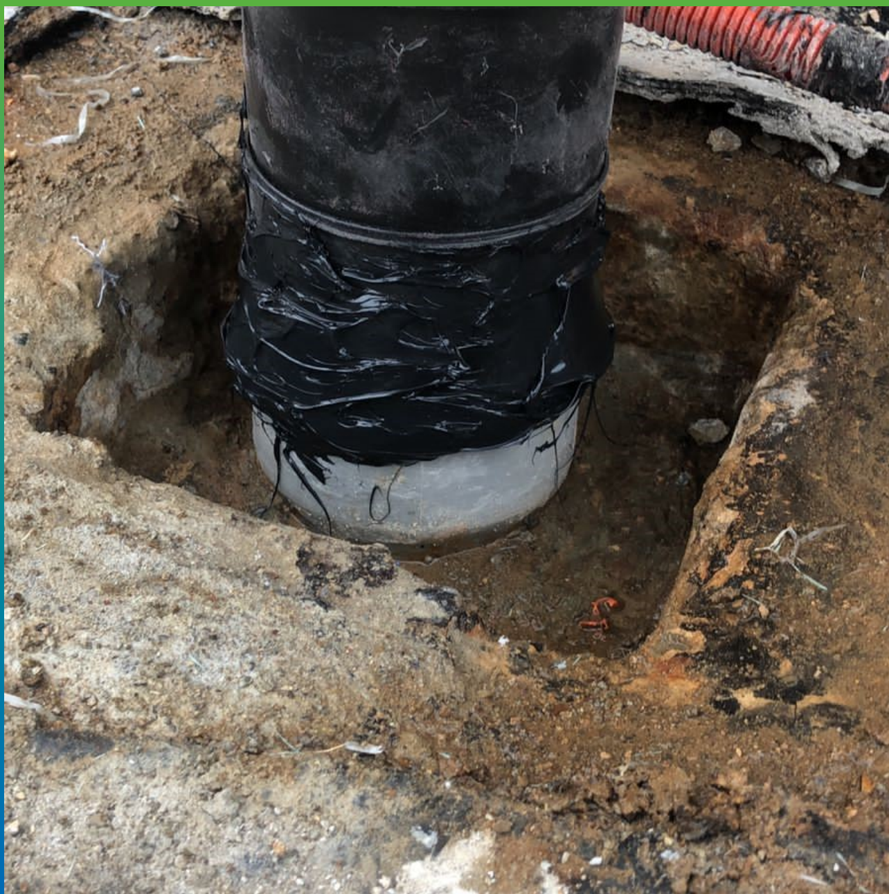
Установка воронки, гидроизолированной составом Манодил Бонд Ф
