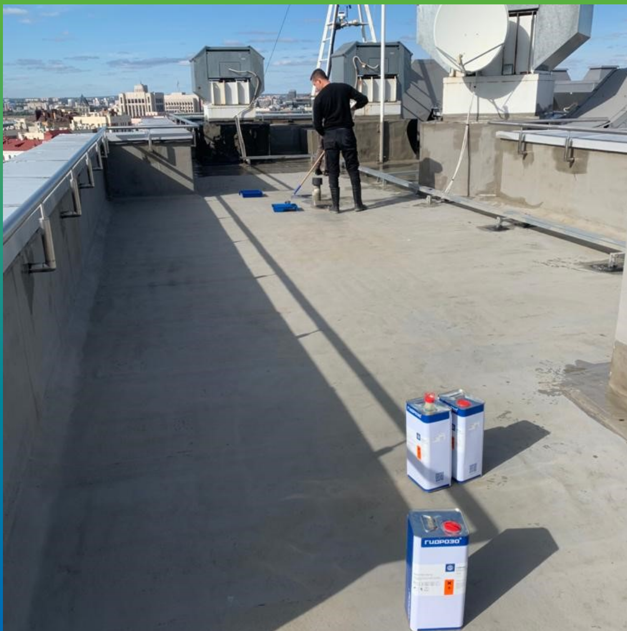
Очистка поверхности перед грунтованием
