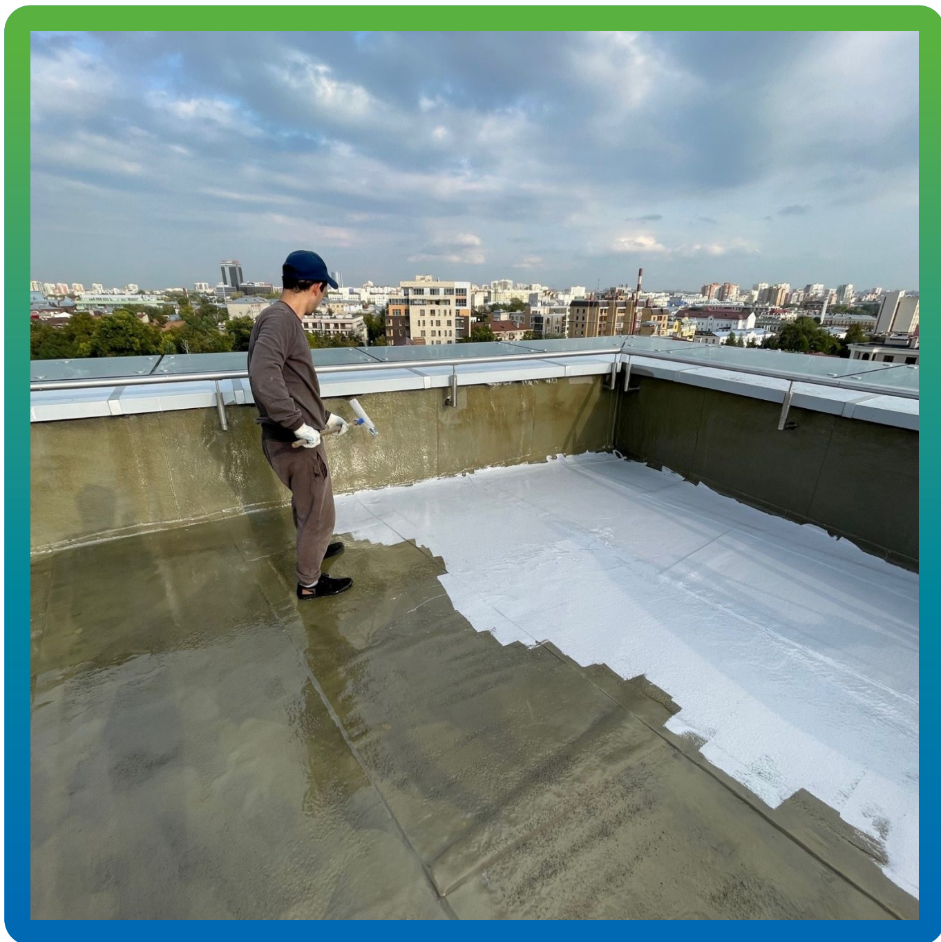
Нанесение материалов системы ДенсТоп
