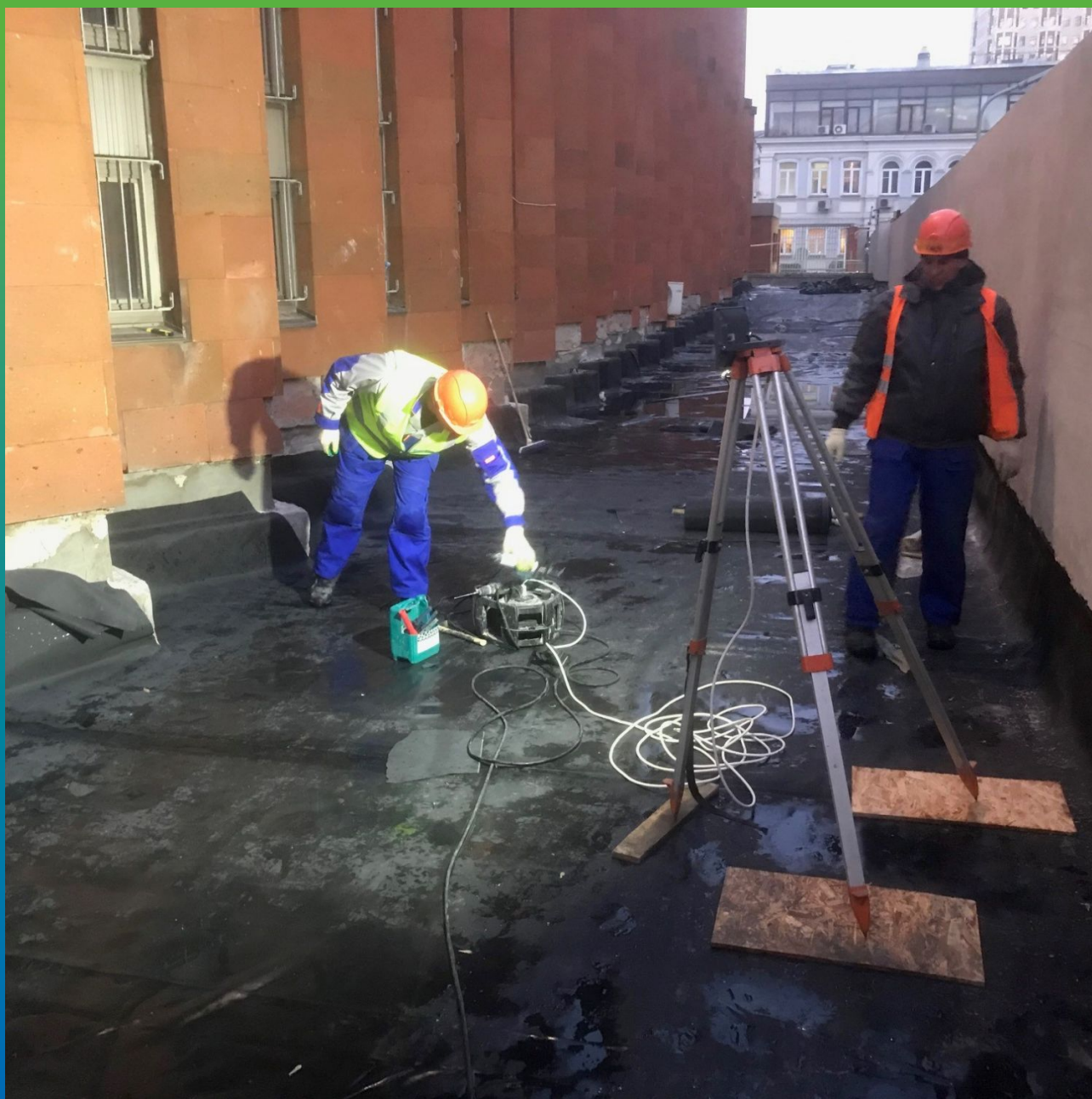
Обварка угловых элементов примыкания к зданию по технологии термобонд
