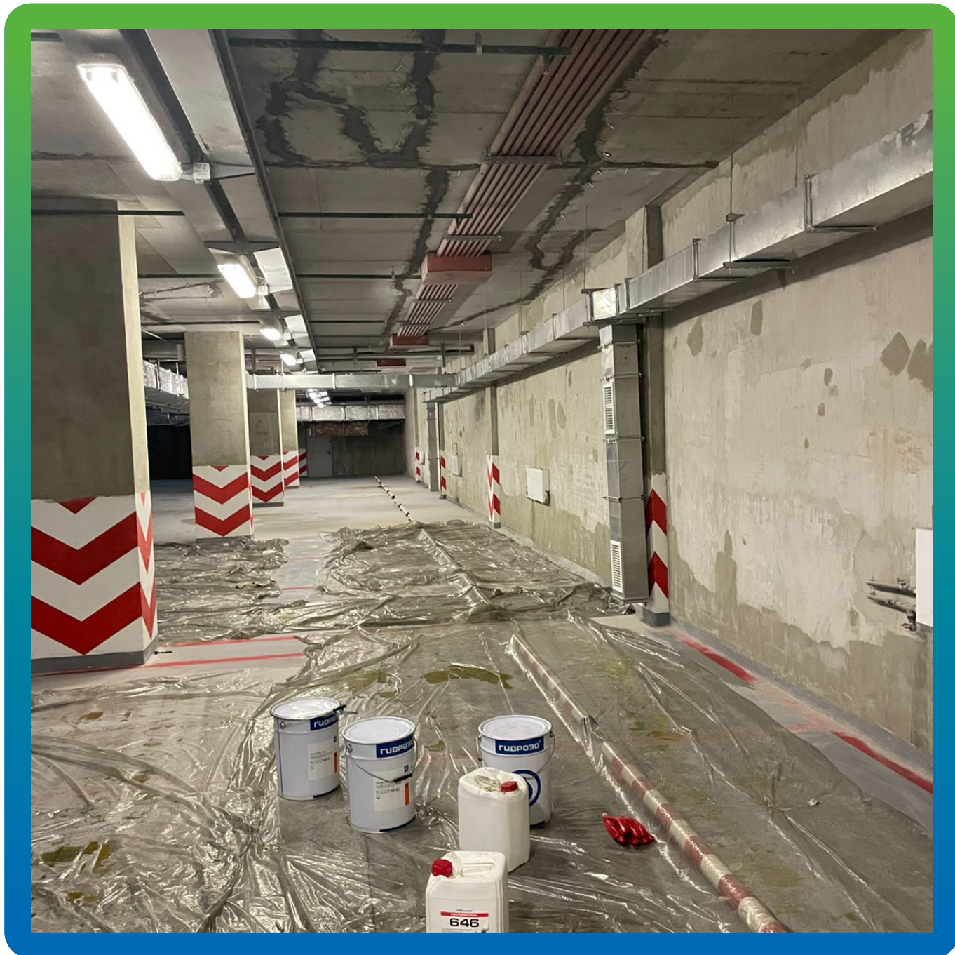
Трещины, проинъектированные составом Манопур 143
