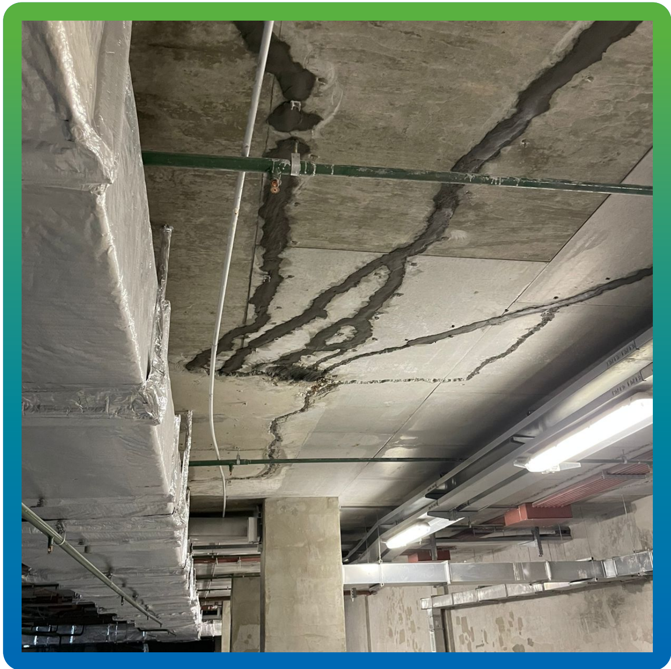
Трещины, зачеканенные составом Стармекс РМЗ
