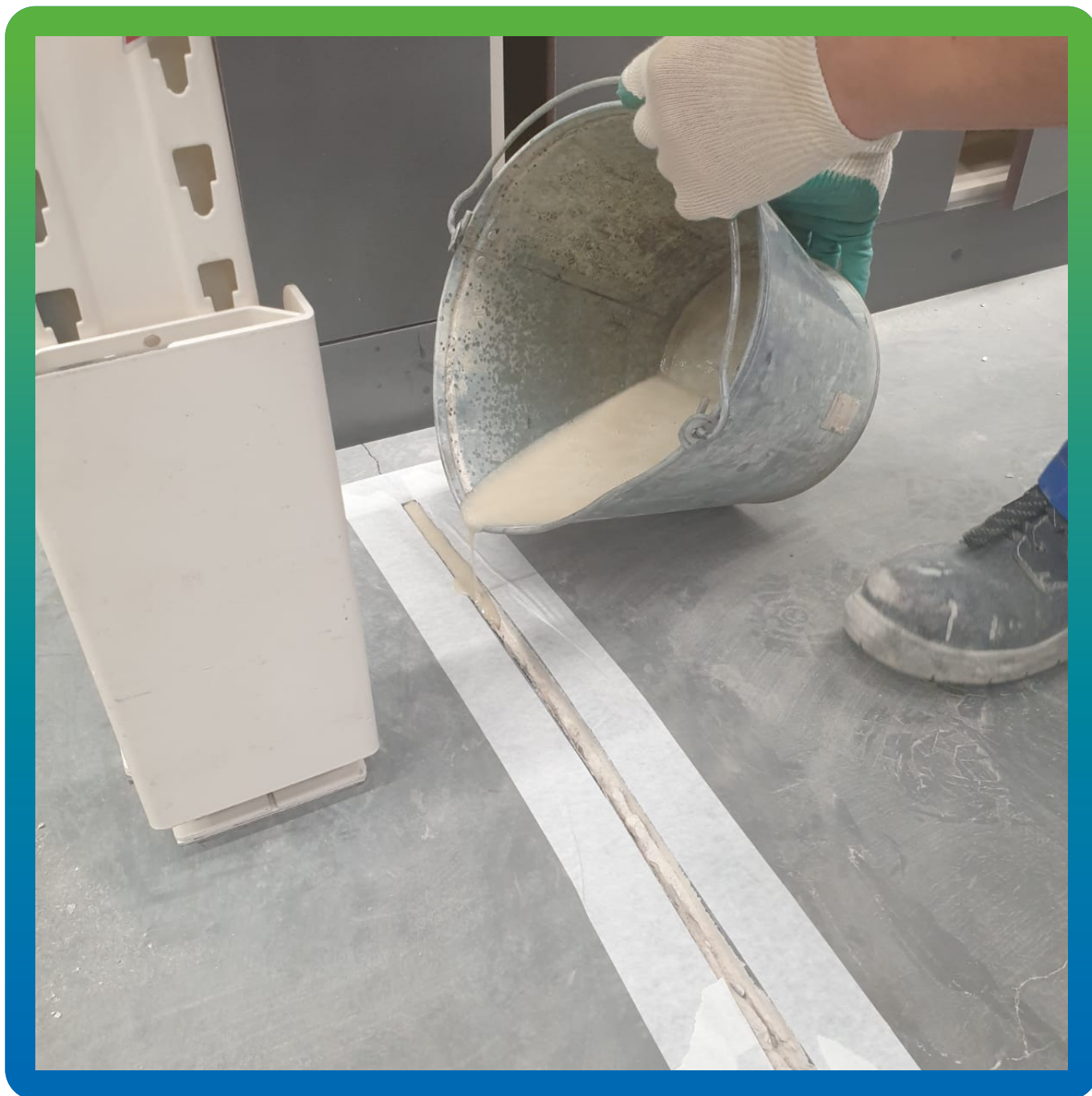
Подача ремонтного состава гравитационным методом
