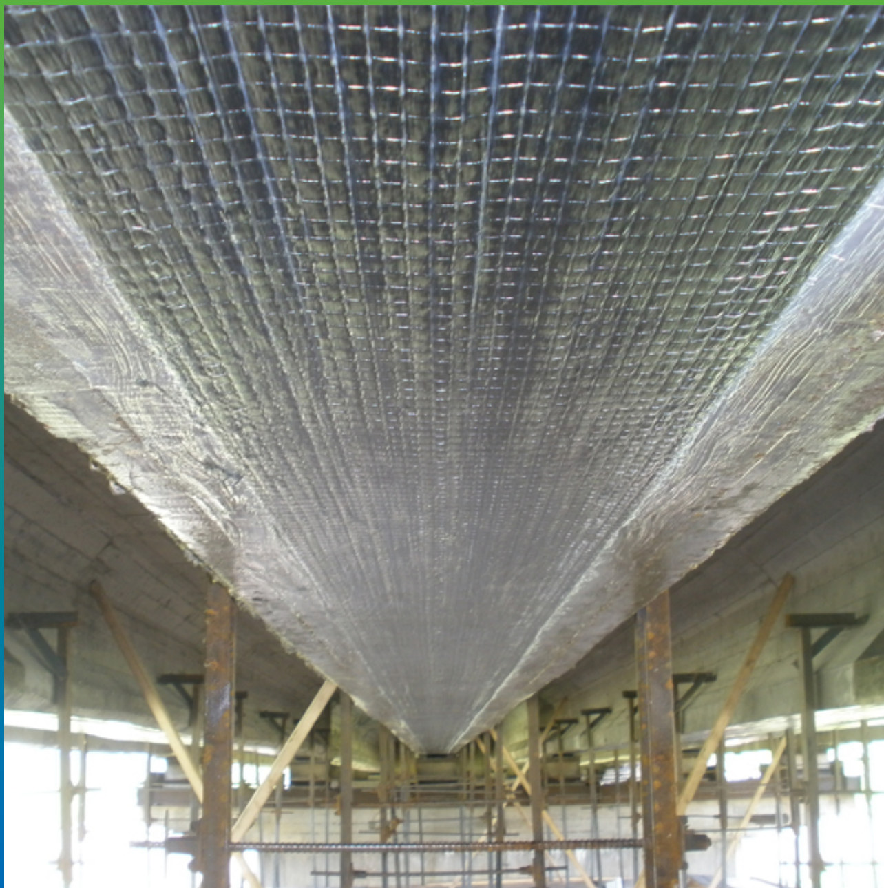
Система усиления Тайфо СЦХ-41 на нижней грани балки
