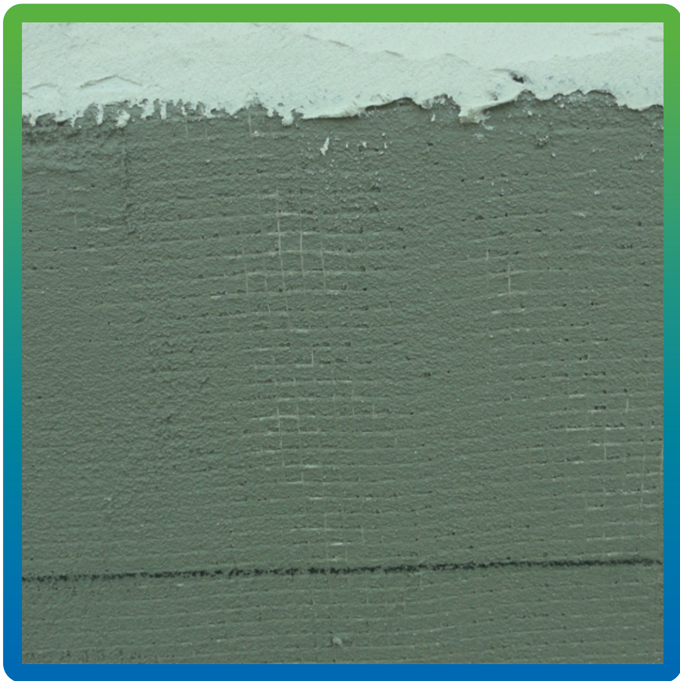
Армирование гидроизоляционного покрытия сеткой
