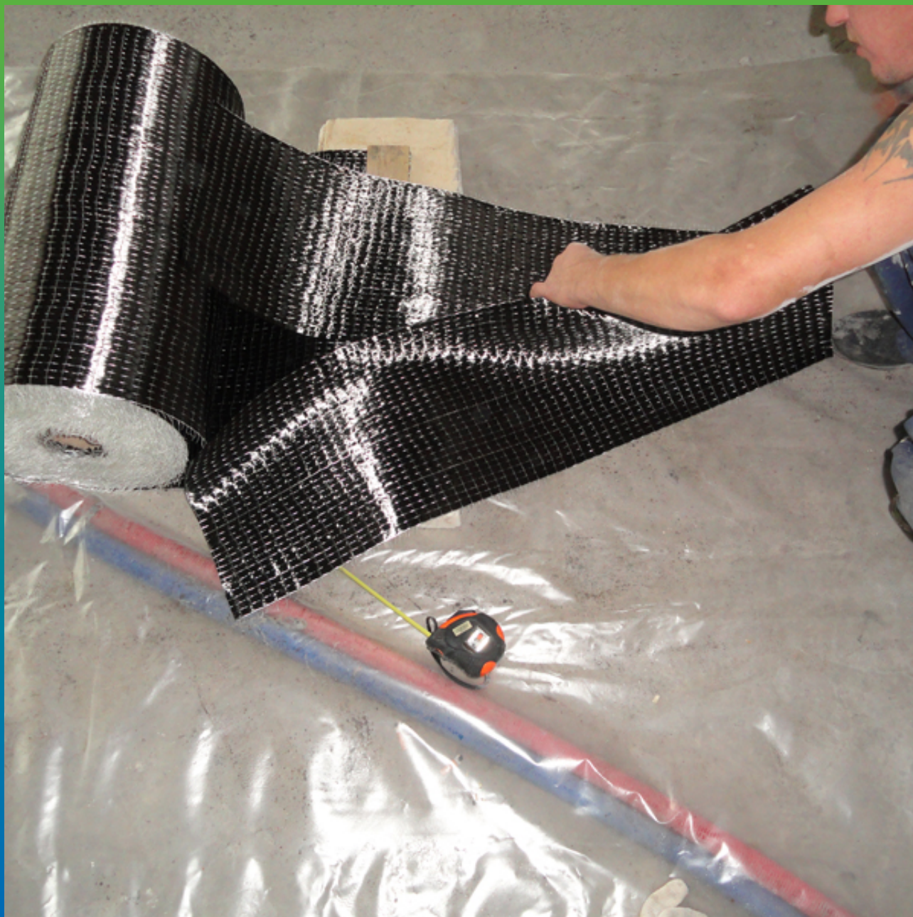
Нарезка холстового материала Тайфо СЦХ-41 перед укладкой
