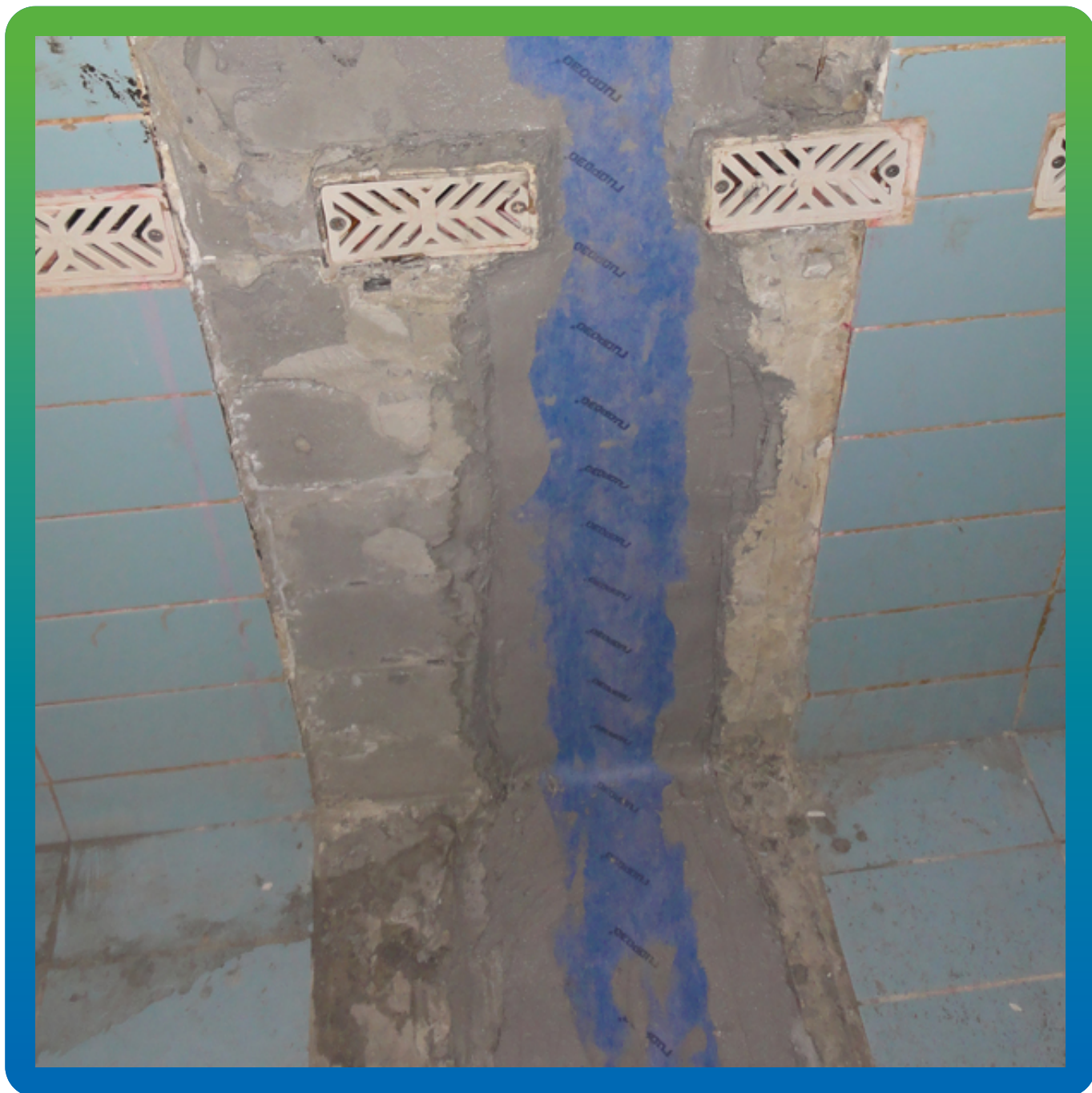
Вид шва, закрытого лентой Манодил Гео на адгезив Манопокс 331
